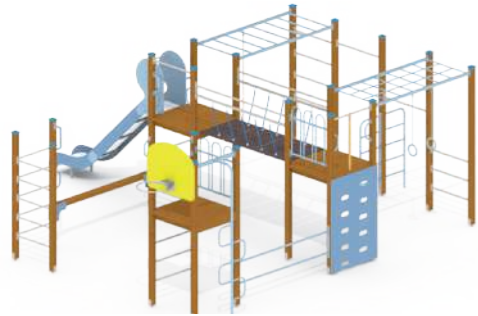
192 244 грн (К) GC-00033 Дитячий спортивний комплекс, 6645x6350x2790мм, висота гірки 1500мм
